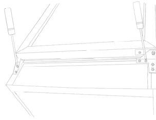
2. Irrota alasarana ja tukipala.
