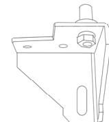
9. Bundhængsel-tappen afmonteres, og bundhængslet vendes 90 grader.
